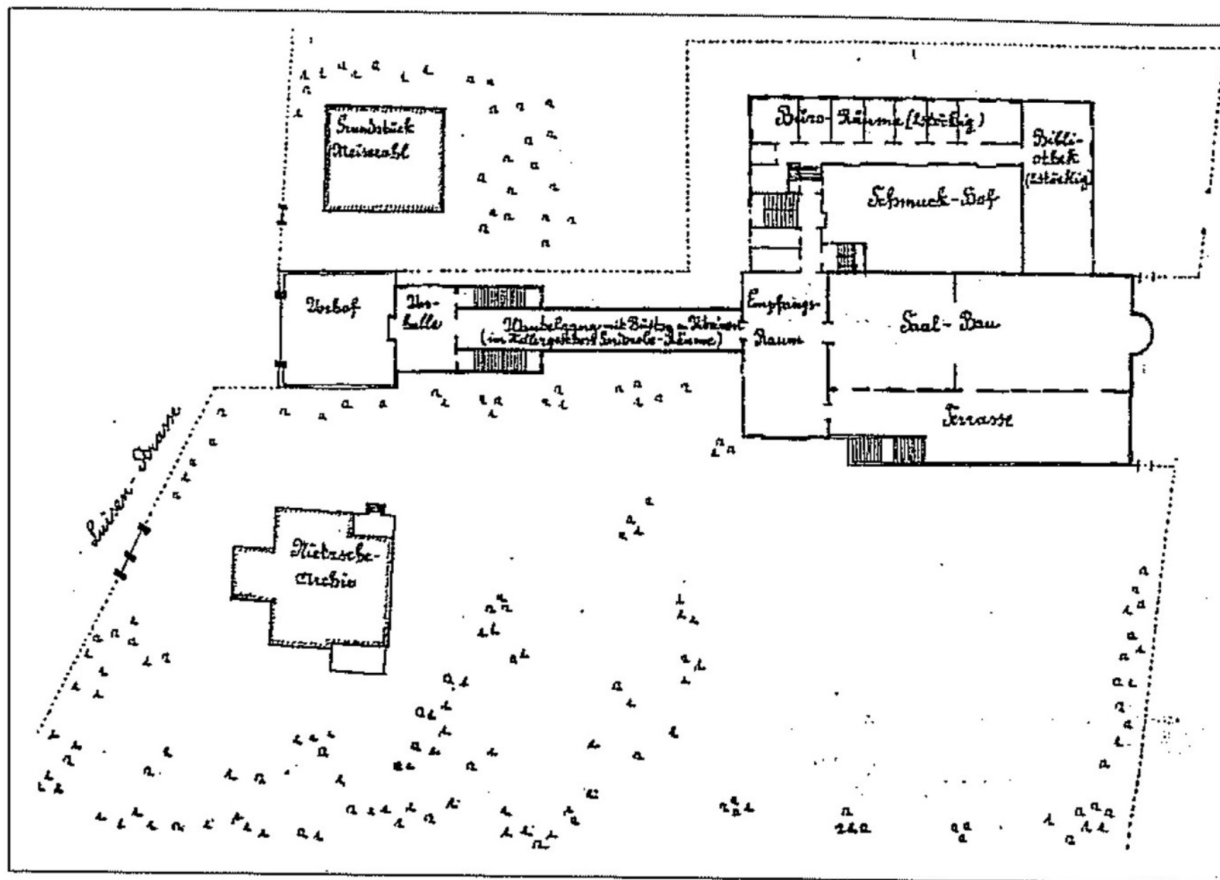
Raumplan Nietzsche-Gedächtnishalle, um 1937
